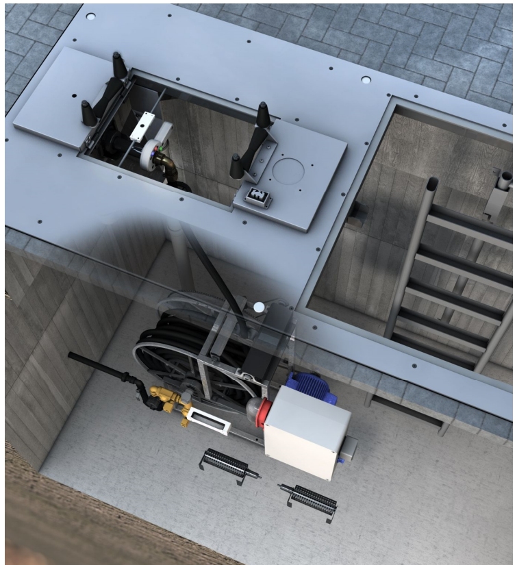
Abb.: Unterflur-Version des Schlauchhaspelsystems easyWinch plus zur Trinkwasserbefüllung
